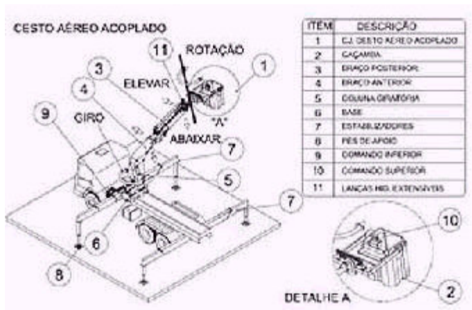
FIGURA 1: EXEMPLO DE ARRANJO COM CESTO ACOPLADO
